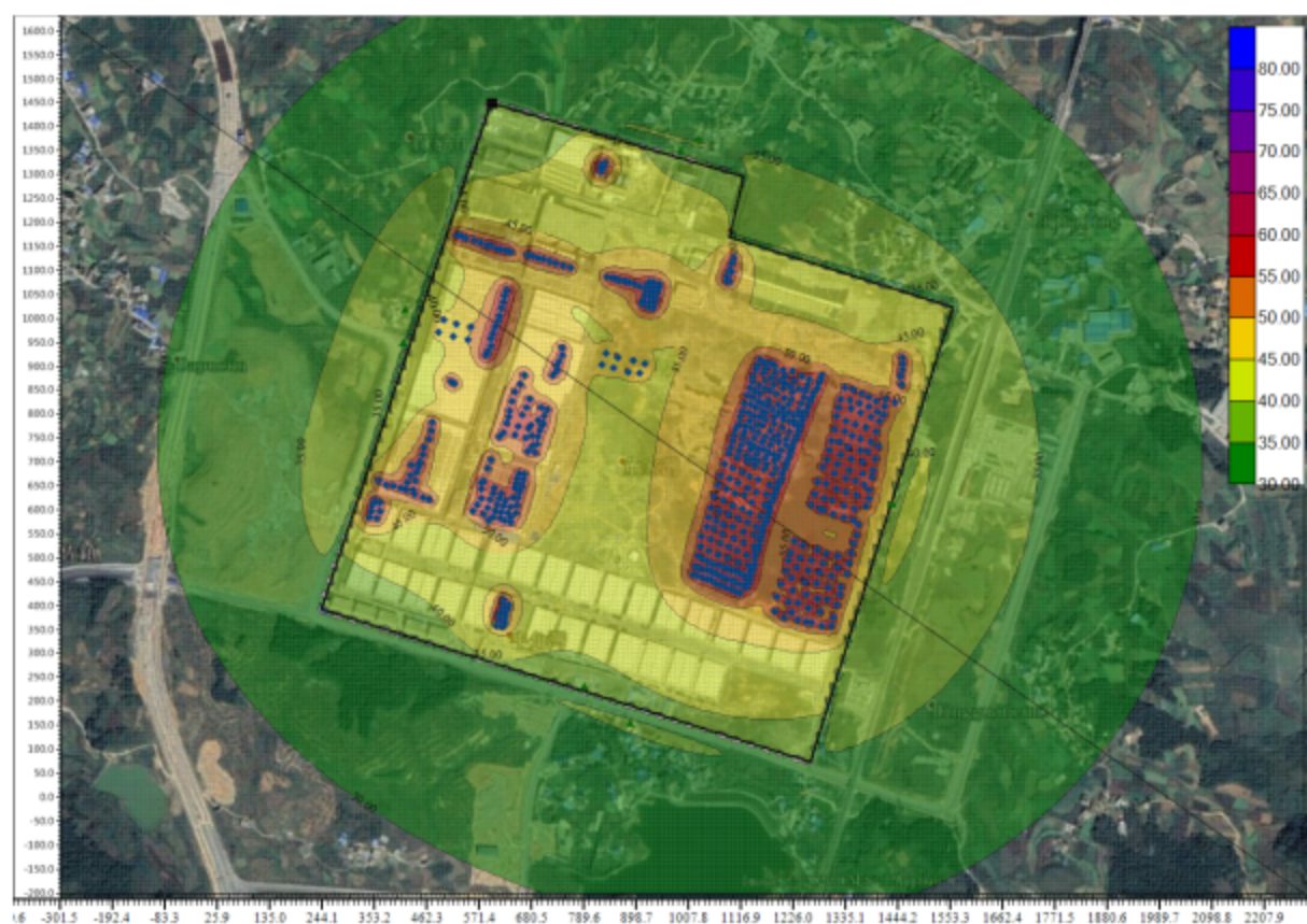
图 4.4-1 运营期等声值线图
