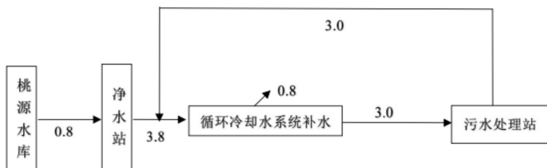
图 2.1-5 本项目水平衡图 单位: \text{m}^3/\text{d}
