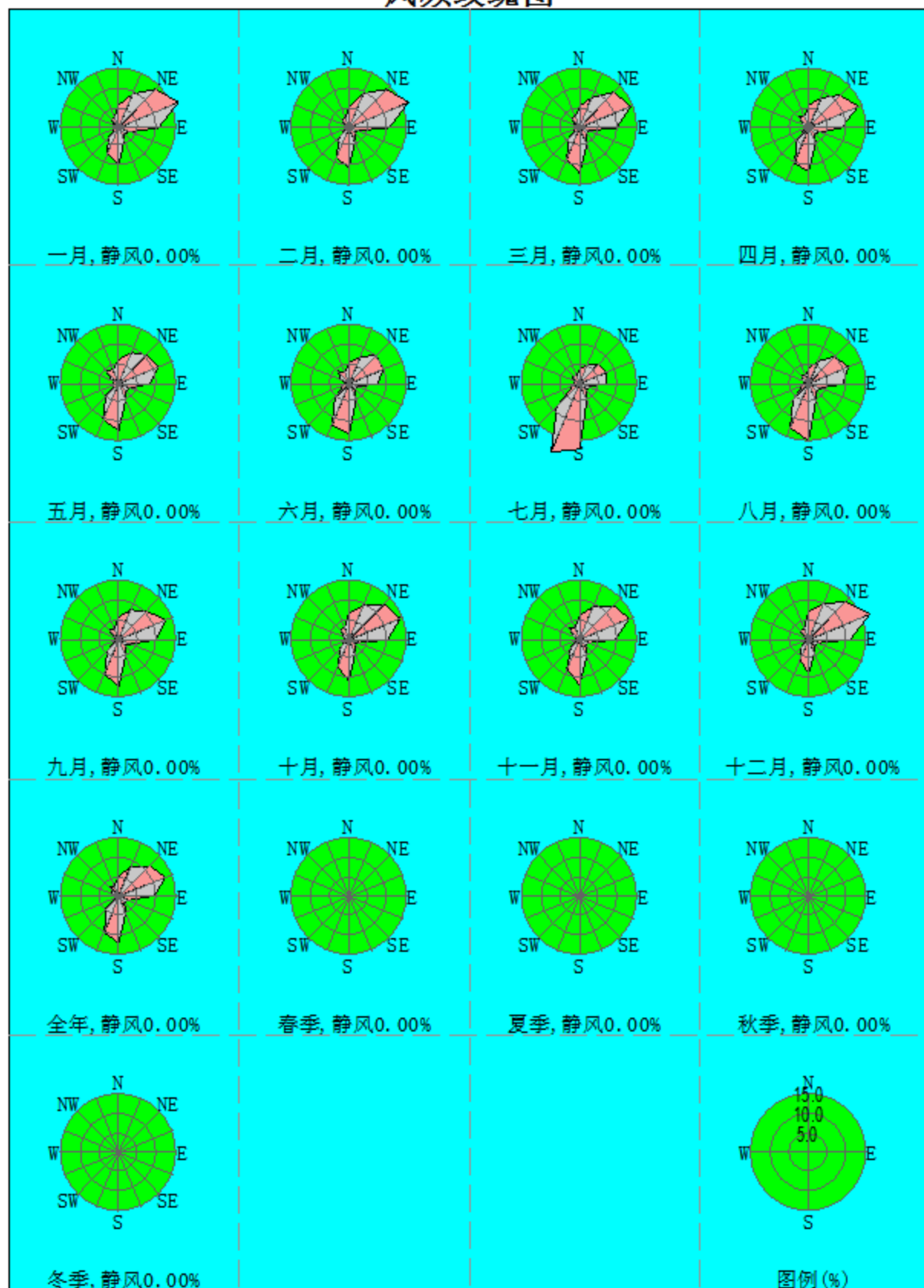
图 4.3-1 修文县 2001-2020 年平均风向频率玫瑰图
